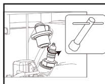
移除火花塞
