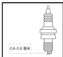
火花塞間隙
