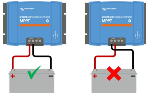
Exemplos de polaridade correta e incorreta (invertida) da bateria
