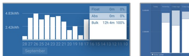
Esquerda: Exemplo de um sistema que passa todo o tempo na fase de carga inicial. Direita: Discriminação das fases de carga - O sistema passa tempo nas fases de carga inicial e absorção.
