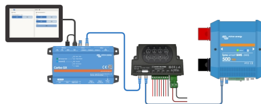
SmartSwitch DC4 ligado
