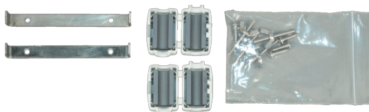
Acessórios incluídos com o GX Touch 50 / 70 Flush
