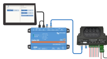
SmartSwitch DC4 conectado na extremidade da rede VE.Can
